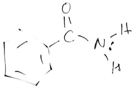
Benzamide
